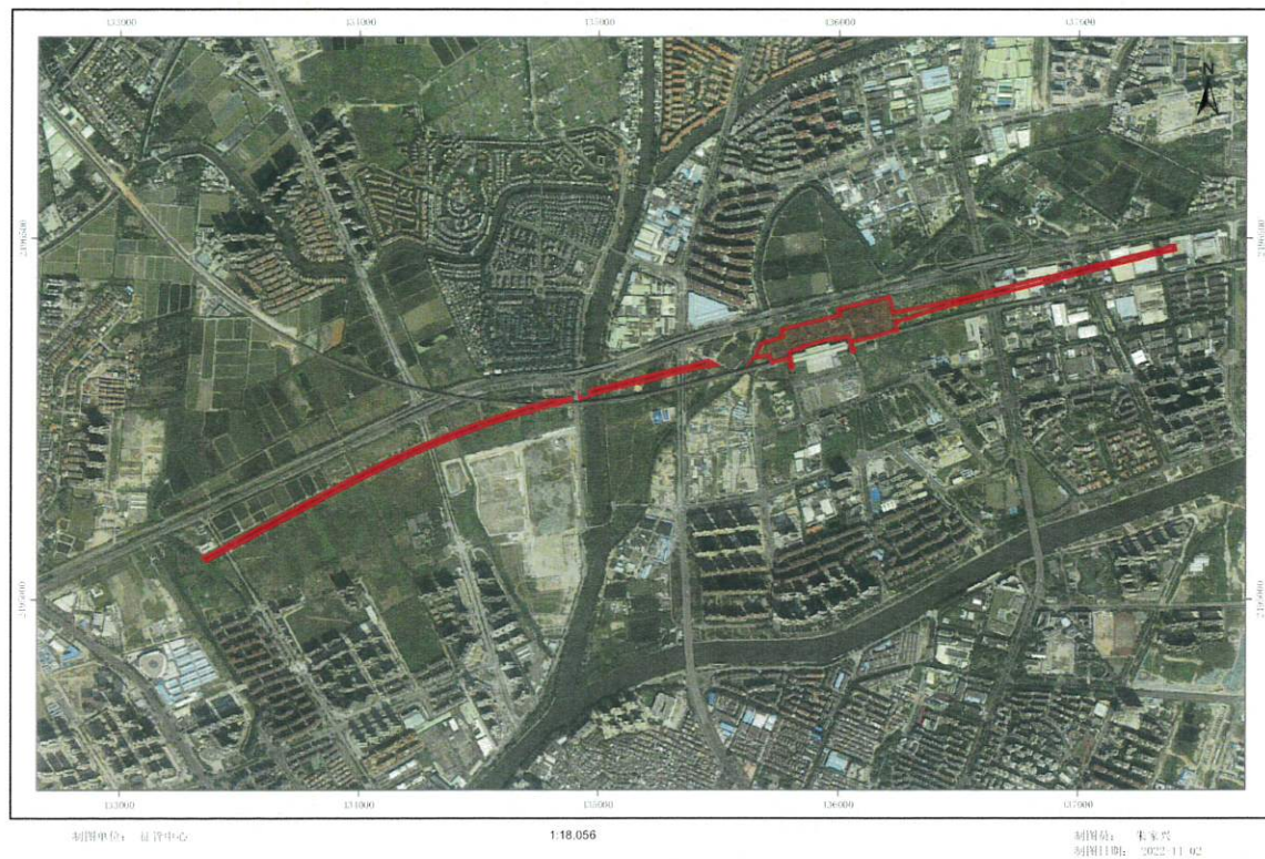
深江铁路项目（石岐街道段）用地红线图
