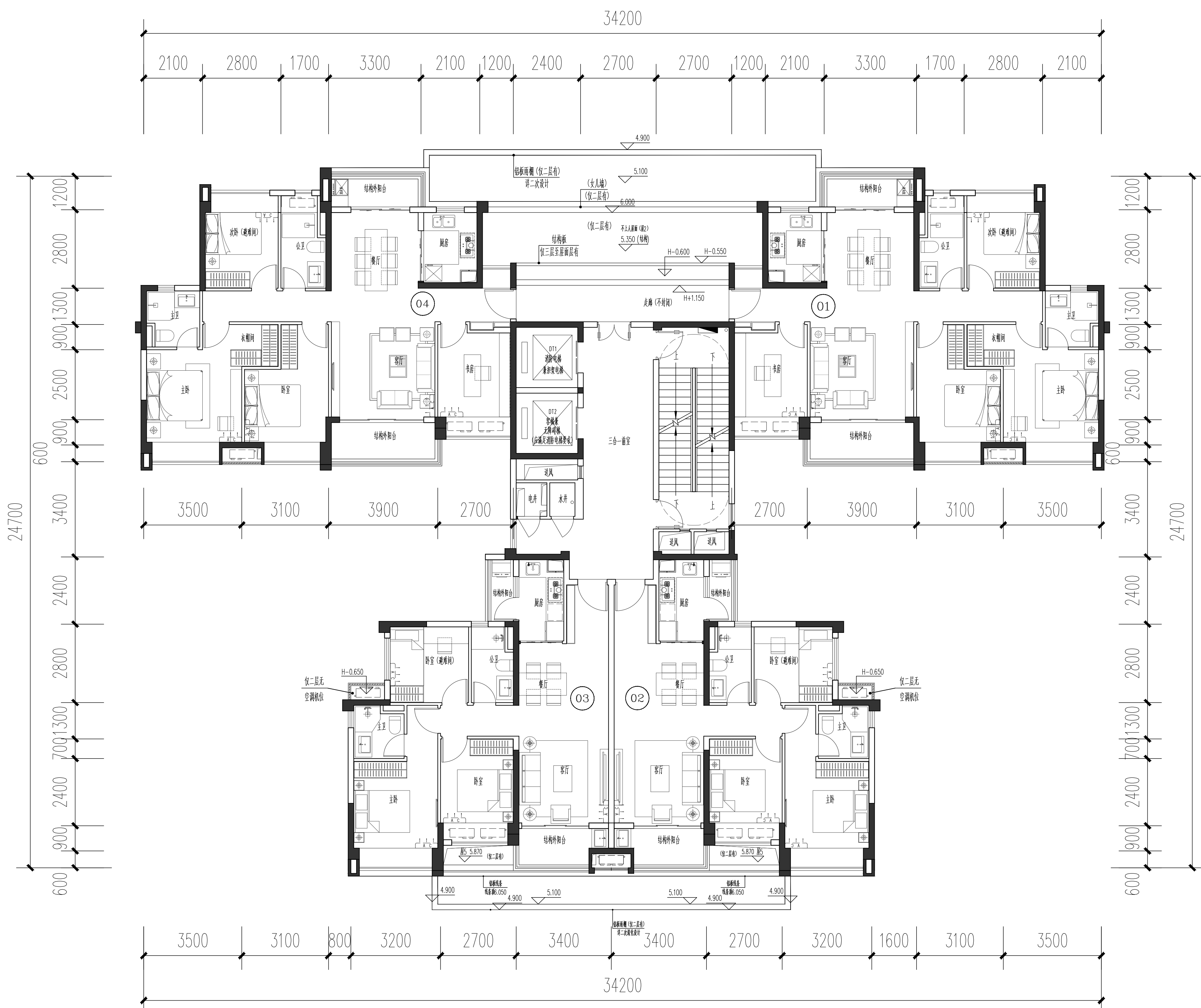
第10栋平面图（2-30层）
