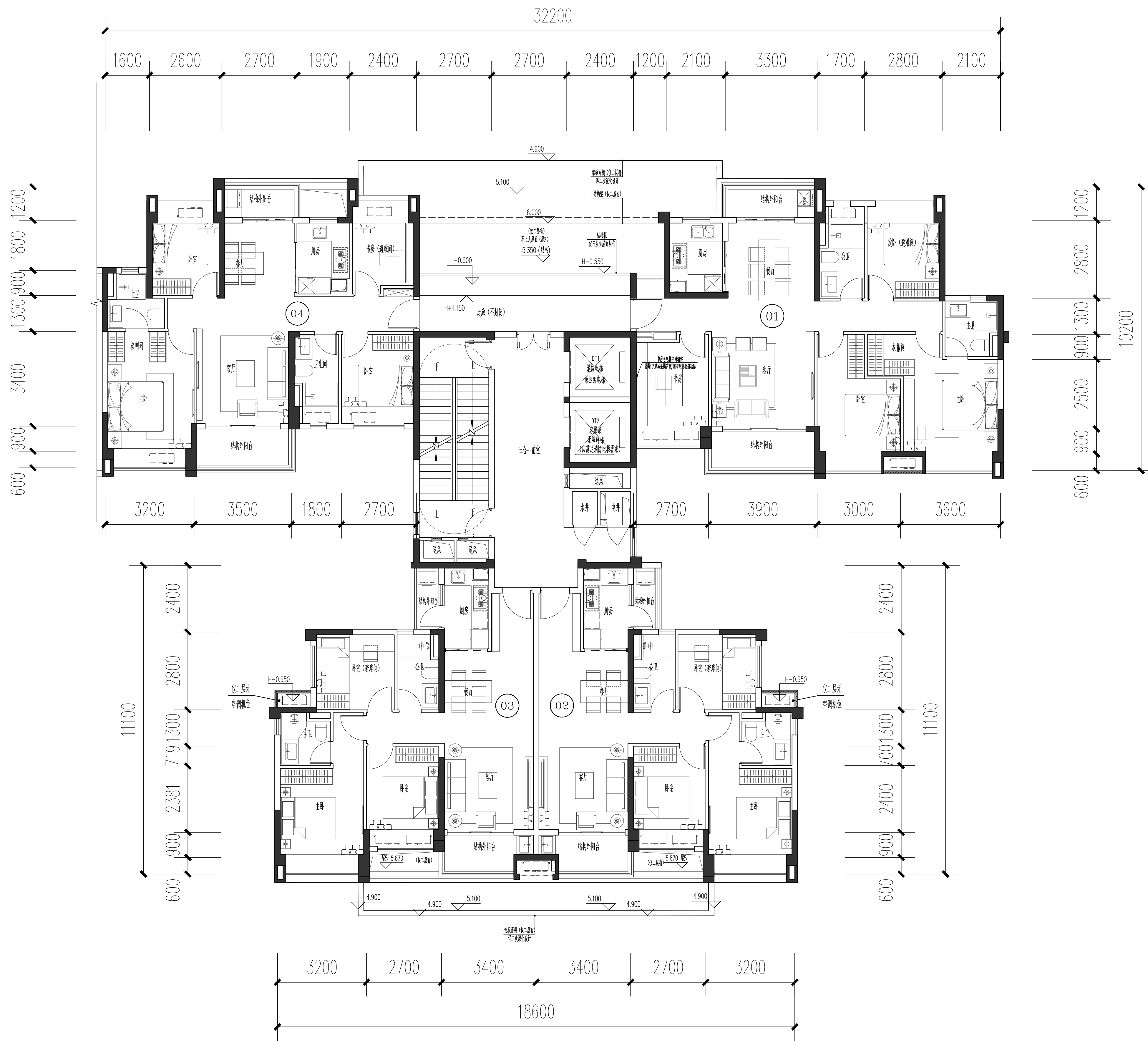
第8栋平面图（2-30层）
