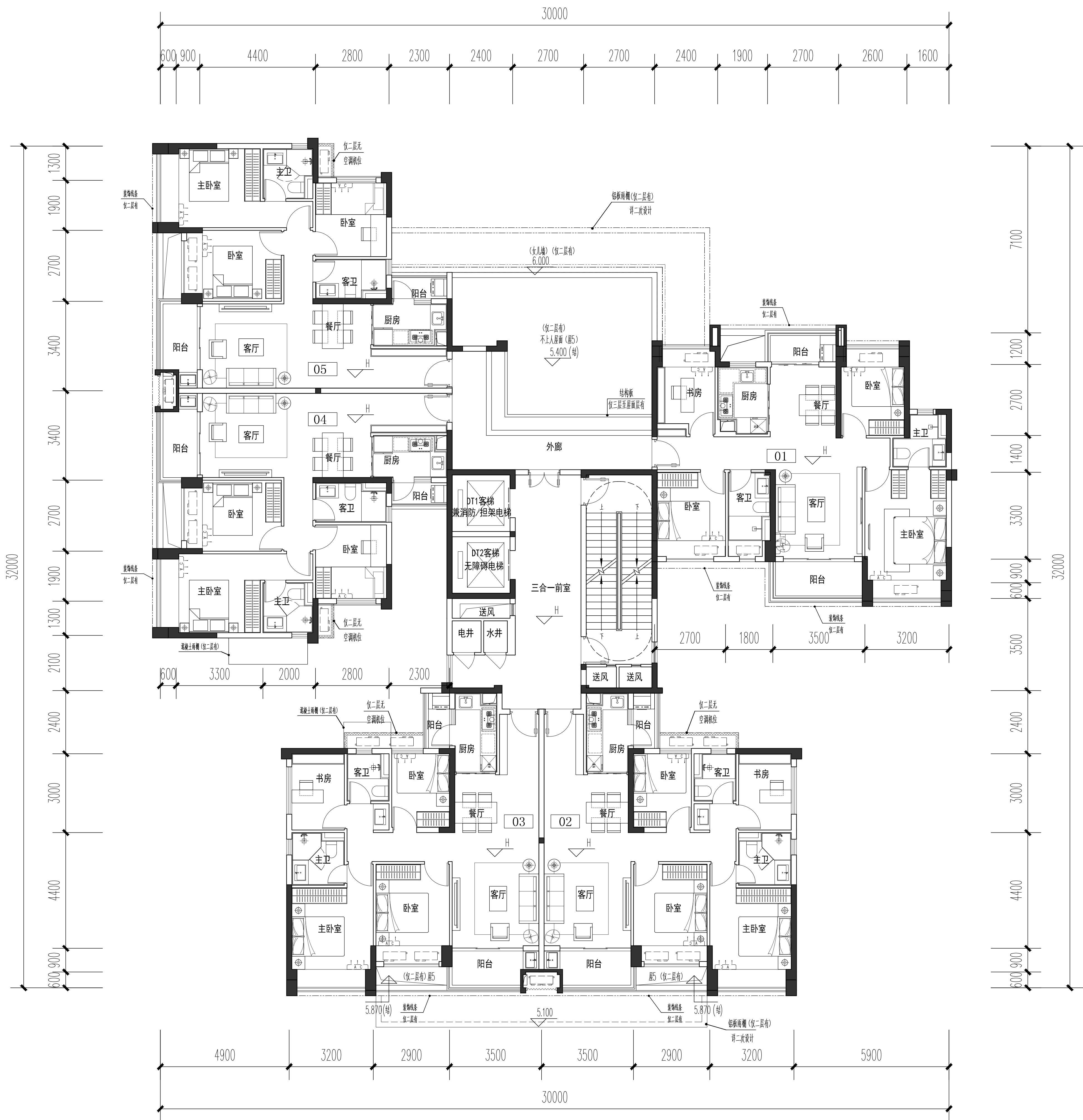
第11栋平面图 (2-31层)
