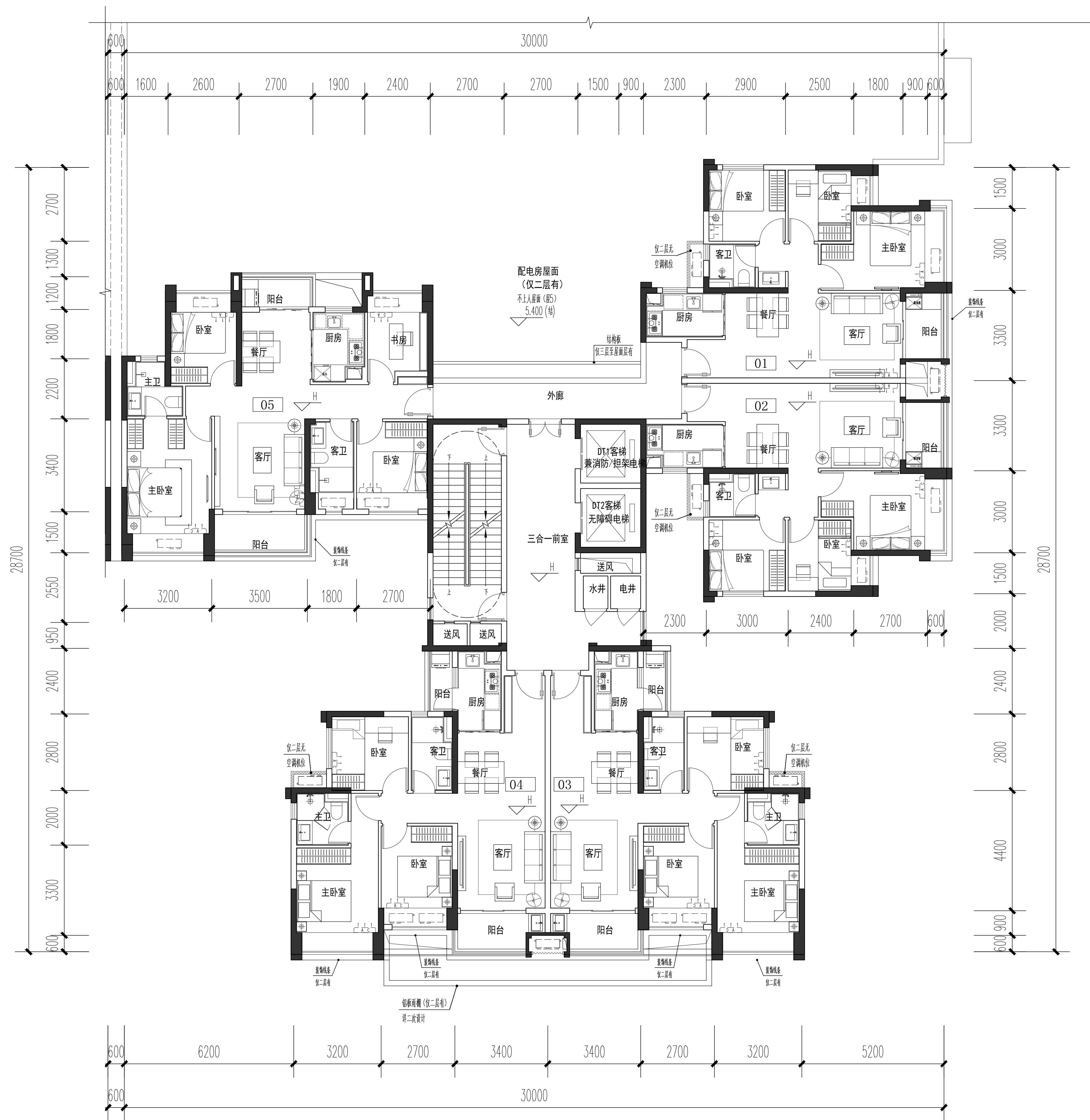
第12栋平面图 (2-32层)
