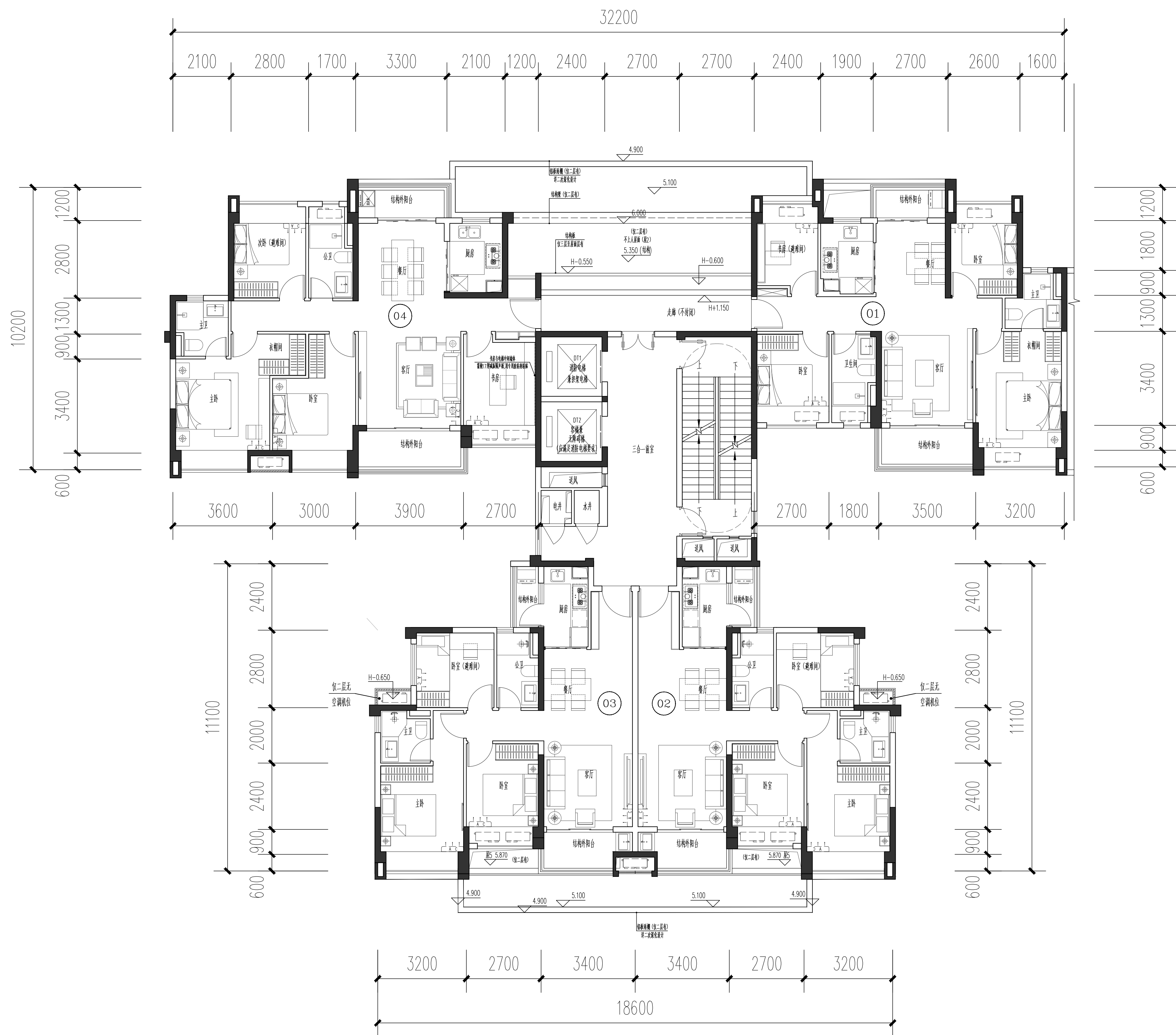
第9栋平面图（2-30层）
