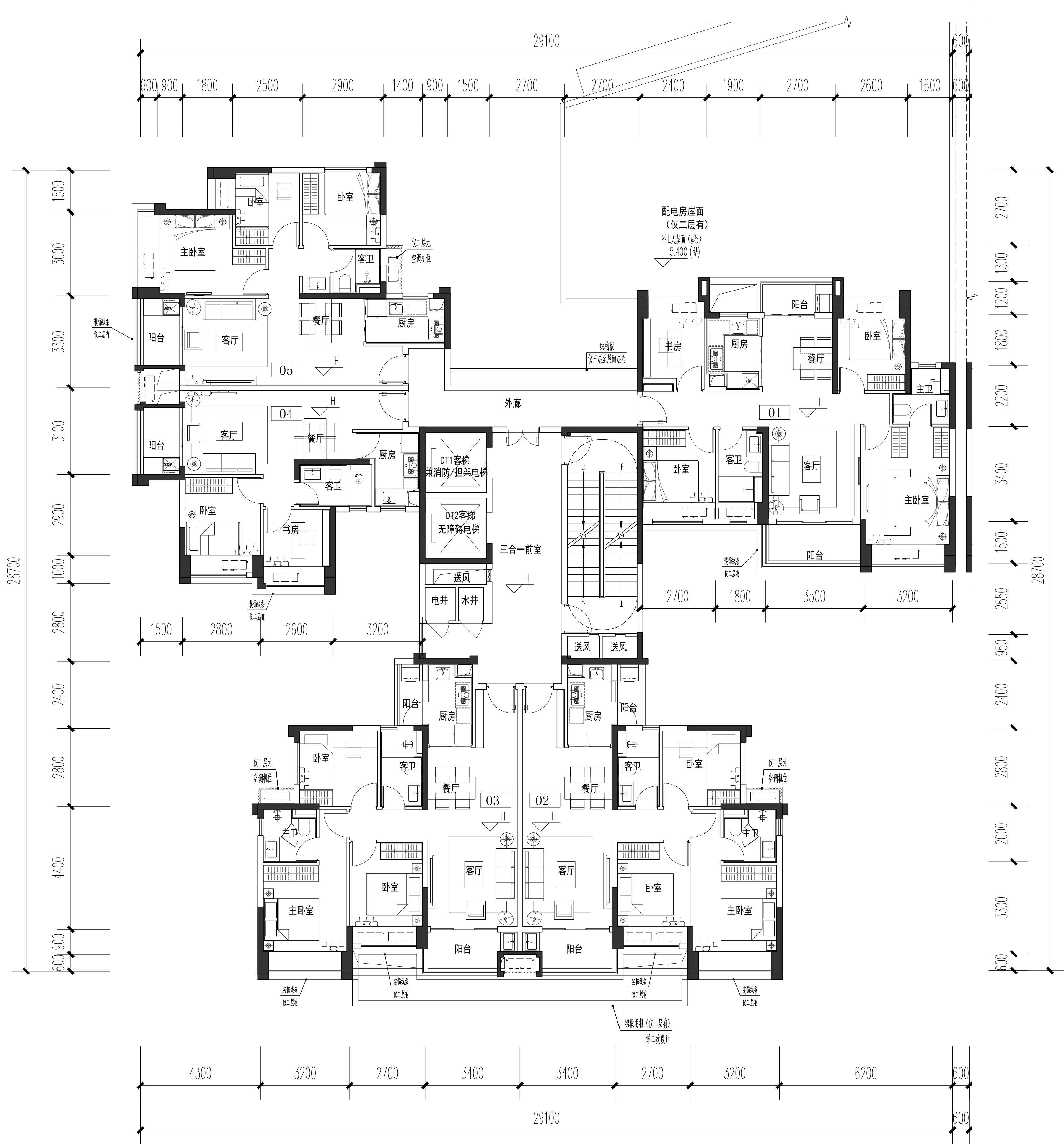
第13栋平面图（2-32层）
