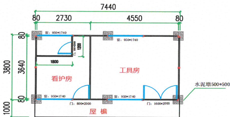
2K*4K*3P(平面图)
